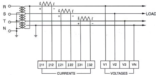
3상4선 Y-Δ 결선(3CT) Mode No 3P4D
