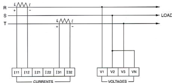
단상3선 결선(2CT) 1P3L Mode No 1P3L
