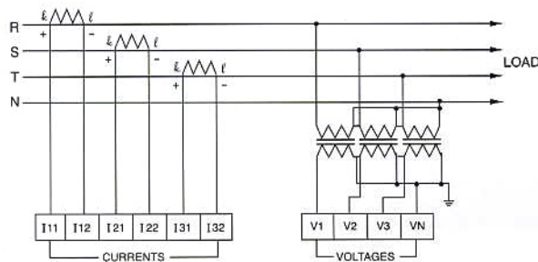
3상4선 Y결선(3PT, 3CT) 3P4L Mode No 3P4L
